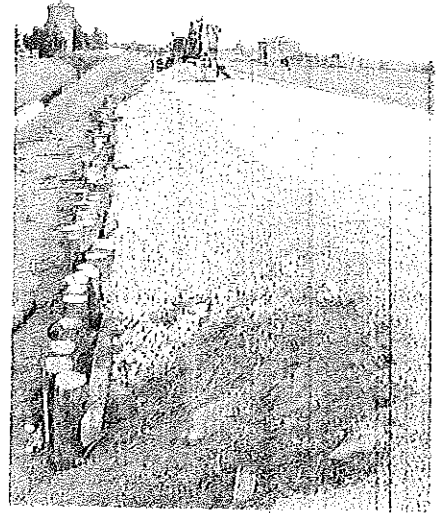
La 'parete' di tronchi realizzata per rinforzare il terrapieno su cui corre la sede stradale tra il ponte della Bastia e Alfonsine
